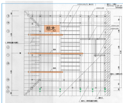
荒井家の2階小屋伏図
